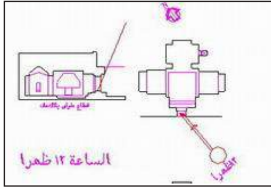
شكل (٣-أ): أشعة الشمس لا تتعدى عتبة مدخل الكهف في الصيف (١٦).
